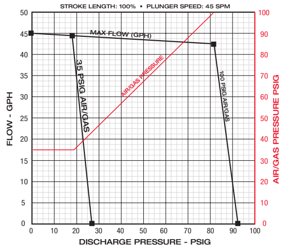
CLD400-316-TFE
