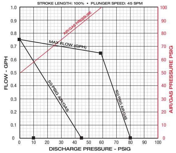
CLD100-316-TFE
