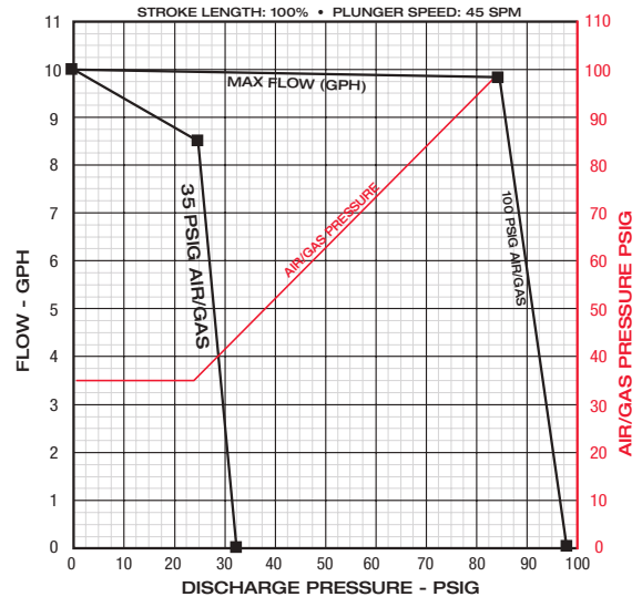
CLD200-316-TFE
