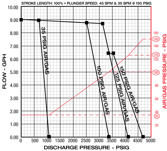
CRP1000V600
